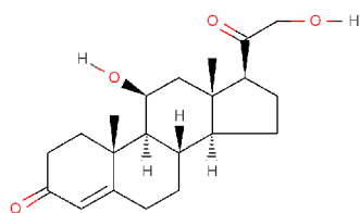
corticosterone
