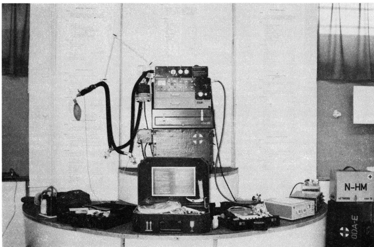
Fotografie 6 Nové typy polních zdravotnických přístrojů: ODA-E, SPIRETA-V
