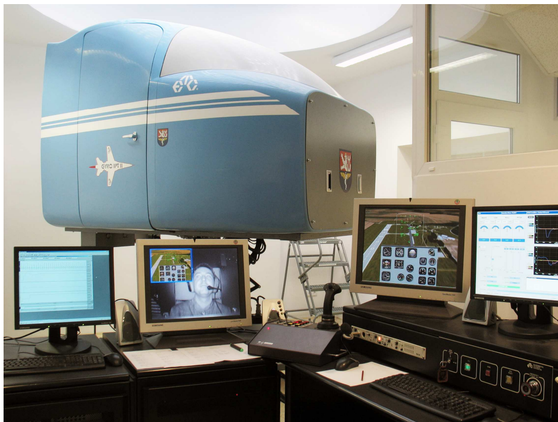
Obr. 5: Dezorientační simulátor GYRO IPT
