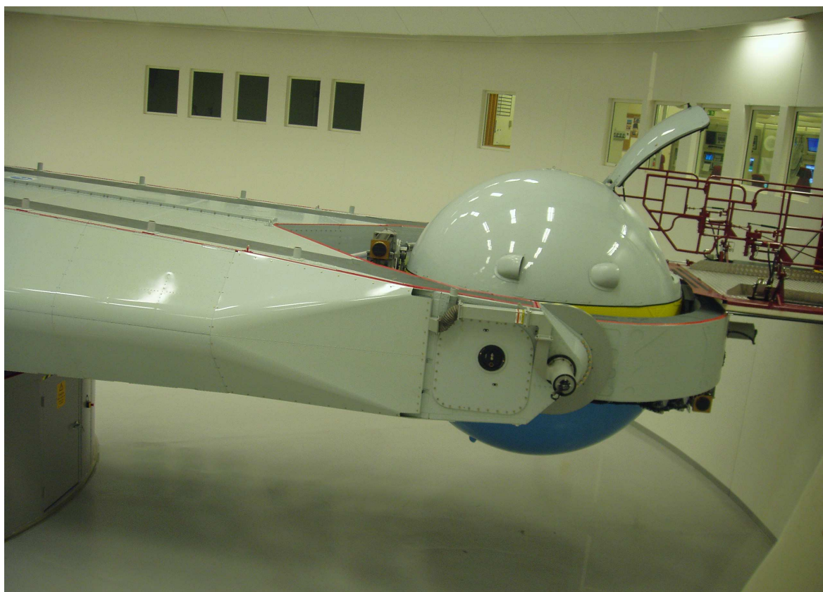
Obr. 4: Lidská centrifuga, Linköping, Švédsko
